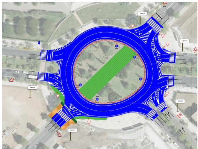
Plano de Planta
